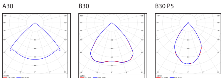
Křivky svítivosti
